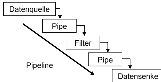
Bild 5-14 Aufbau einer Pipeline beim Muster Pipes and Filters
