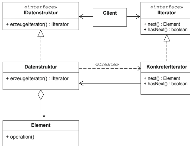
Bild 4-56 Klassendiagramm des Iterator-Masters
