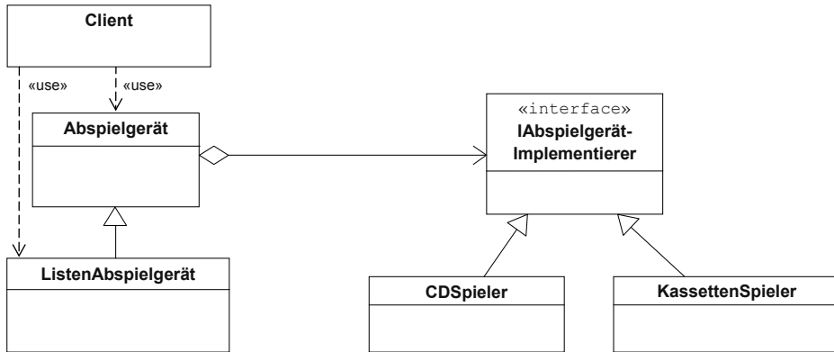
Bild 4-6 Klassendiagramm für das Beispiel
