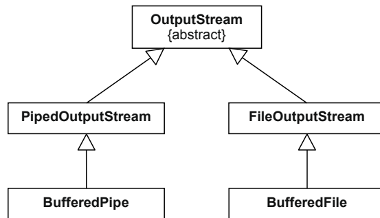
Bild 4-14 Erweiterung von Funktionalität durch Ableiten
