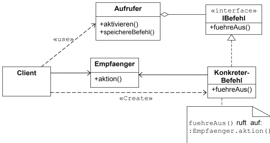
Bild 4-30 Klassendiagramm des Befehlsmasters
