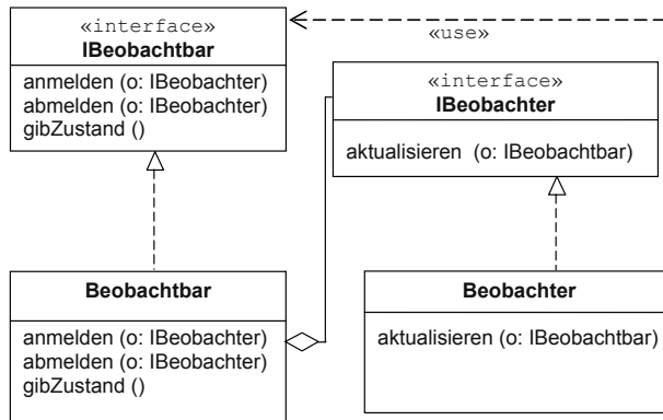
Bild 1-14 Klassendiagramm des Beobachter-Entwurfsmusters
