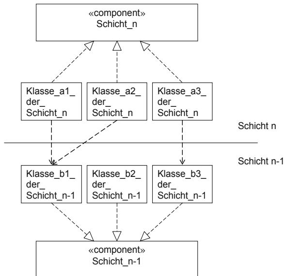
Bild 5-3 Beispiel für die Abhängigkeitsbeziehung zwischen Objekten benachbarter Komponenten
