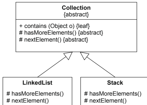
Bild 4-29 Container-Klassen zur Veranschaulichung der Schablonenmethode
