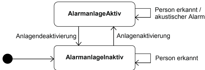
Bild 4-44 Zustandsdiagramm für die Alarmanlage
