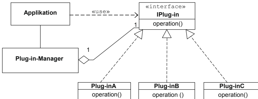
Bild 5-22 Klassendiagramm einer Plug-in-Architektur mit einem einzigen Interface
