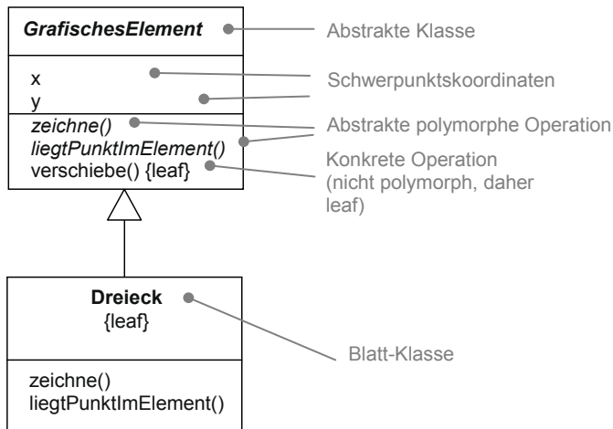
Bild 1-9 Die abstrakte Klasse GrafischesElement als symbolisches Framework
