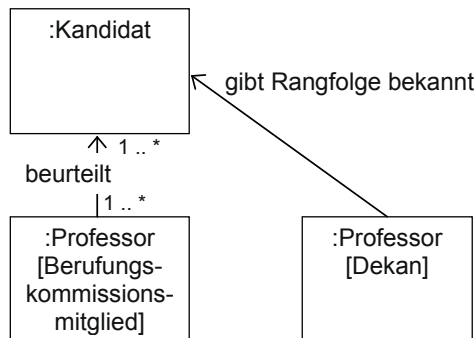
Bild 4-46 Rollen in einem Objektdiagramm
