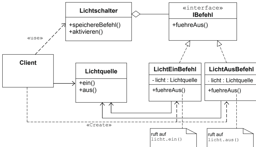
Bild 4-32 Klassendiagramm zum Programmbeispiel Befehlsmuster
