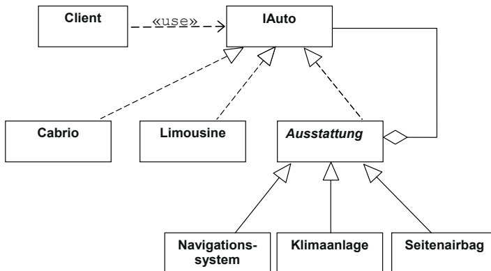
Bild 4-12 Klassendiagramm des Programmbeispiels zum Dekorierer
