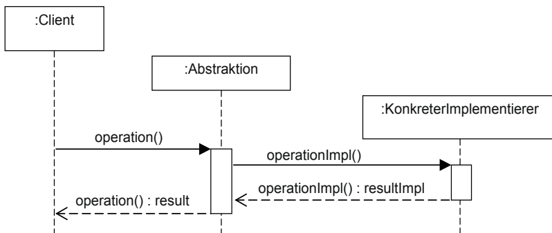
Bild 4-5 Sequenzdiagramm des Brücke-Musters
