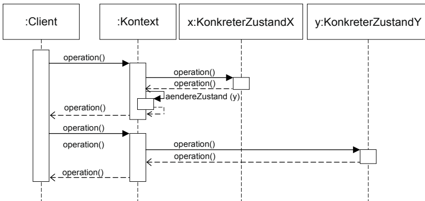
Bild 4-43 Sequenzdiagramm des Entwurfsmusters Zustand
