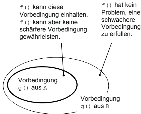
Bild 1-7 Aufweichen einer Vorbedingung in einer abgeleiteten Klasse
