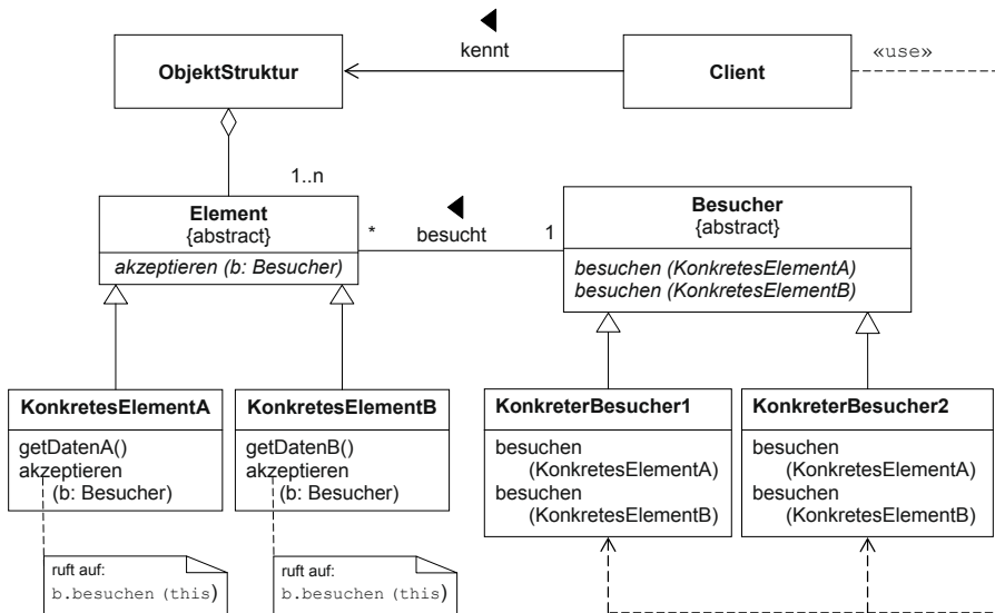
Bild 4-53 Klassendiagramm des Besucher-Musters unter Verwendung einer Objektstruktur
