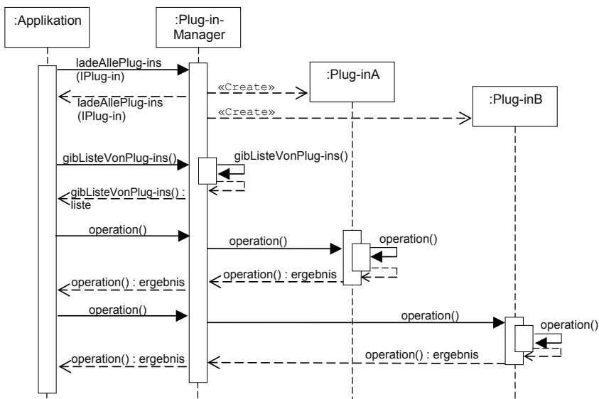
Bild 5-23 Sequenzdiagramm eines typischen Systems nach der Plug-in-Architektur
