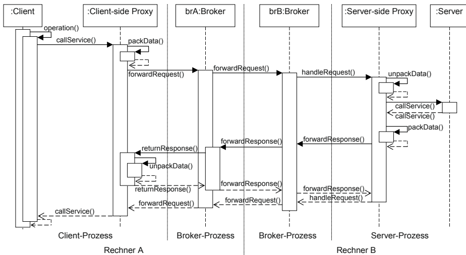
Bild 5-26 Dynamischer Ablauf mit mehreren Brokern
