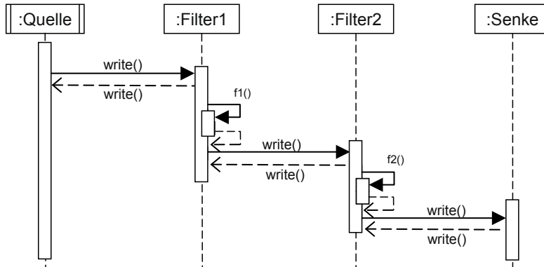
Bild 5-17 Sequenzdiagramm für das Push-Prinzip
