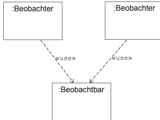
Bild 4-33 Abhängigkeit eines Beobachters vom beobachtbaren Objekt
