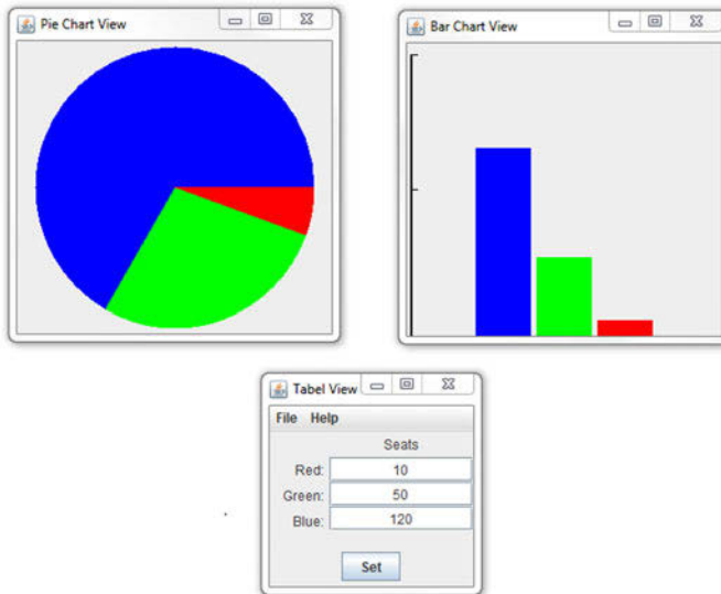
Bild 5-45 Beispielprogramm für das MVC-Architekturmuster
