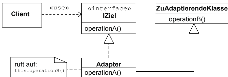
Bild 4-1 Klassendiagramm Klassen-Adapter
