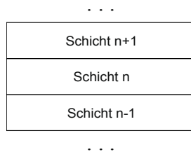
Bild 5-1 Schichtenmodell
