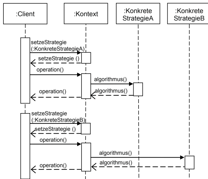
Bild 4-37 Sequenzdiagramm Strategie
