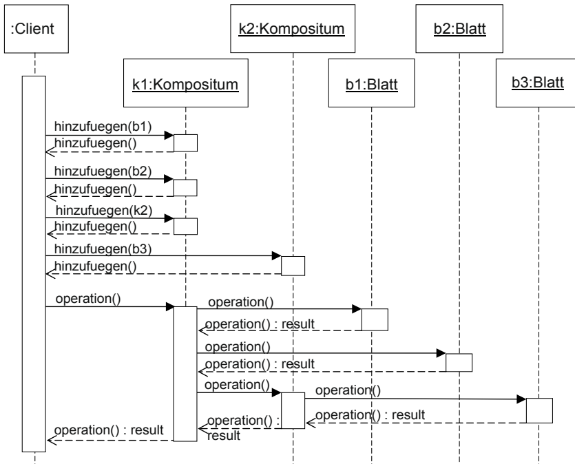
Bild 4-22 Sequenzdiagramm Kompositum-Muster
