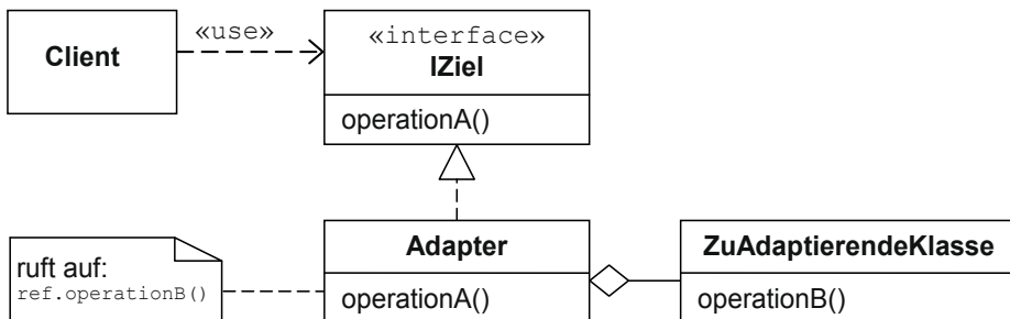
Bild 4-2 Klassendiagramm Objekt-Adapter
