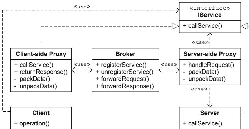
Bild 5-24 Klassendiagramm Broker-Muster
