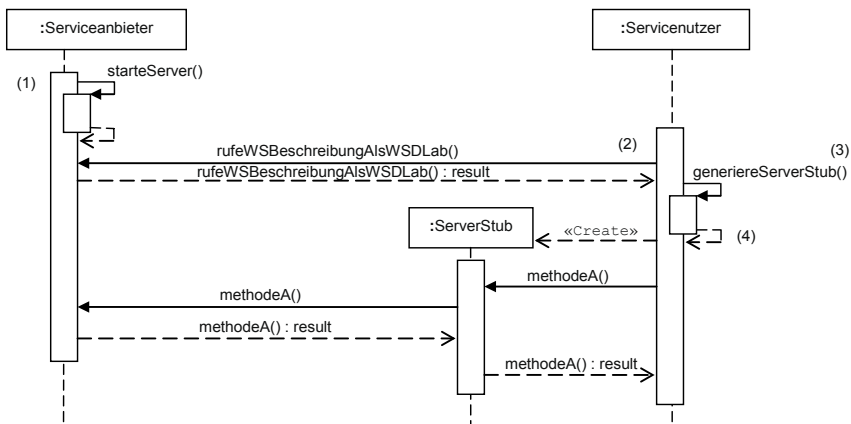
Bild 5-34 JAX-WS Sequenzdiagramm
