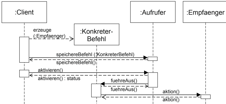
Bild 4-31 Sequenzdiagramm des Befehlsmodells
