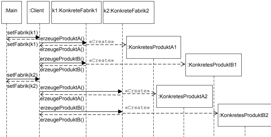
Bild 4-61 Sequenzdiagramm des Musters Abstrakte Fabrik
