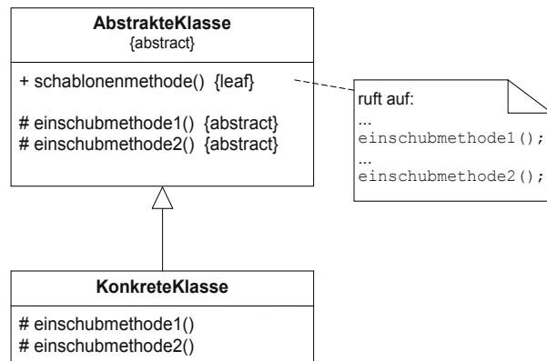
Bild 4-27 Beispiel für ein Klassendiagramm der Schablonenmethode
