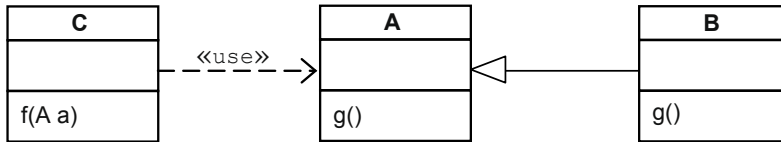
Bild 1-6 Überschreiben einer Methode
