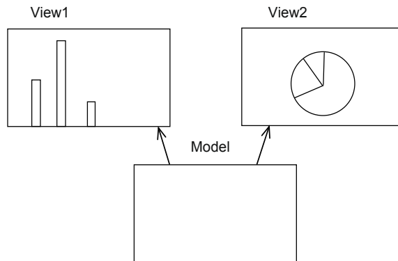
Bild 5-39 Aktualisierung zweier Views durch das Model
