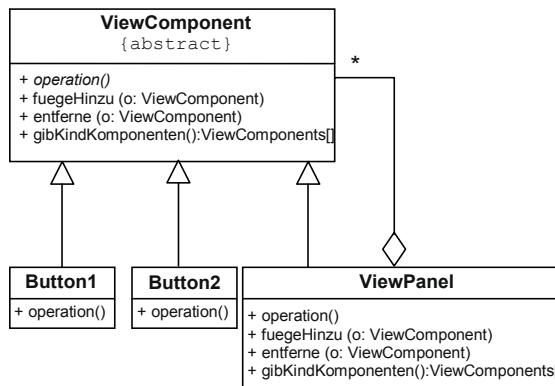
Bild 5-42 Klassendiagramm Kompositum-Muster im MVC
