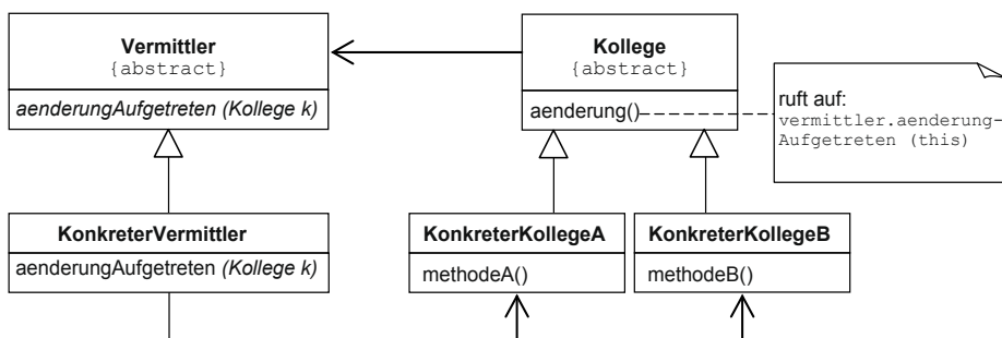
Bild 4-40 Klassendiagramm des Vermittler-Musters
