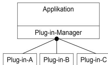
Bild 5-21 Konzept einer Plug-in-Architektur
