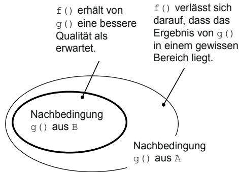
Bild 1-8 Verschärfen einer Nachbedingung in einer abgeleiteten Klasse
