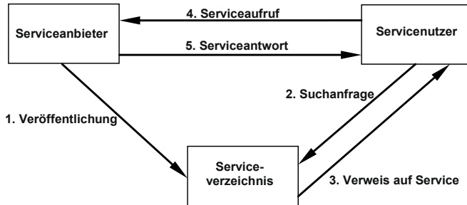
Bild 5-30 Zusammenarbeit in einer SOA
