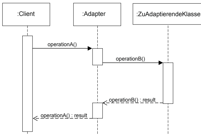
Bild 4-3 Sequenzdiagramm des Adapter-Musters
