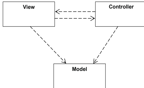
Bild 5-38 Komponenten der MVC-Architektur und ihre Abhängigkeiten
