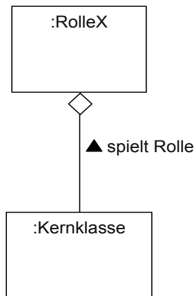
Bild 4-47 Objektdiagramm des Rollen-Musters
