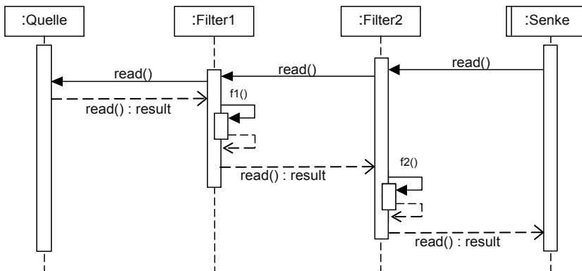
Bild 5-16 Sequenzdiagramm für das Pull-Prinzip
