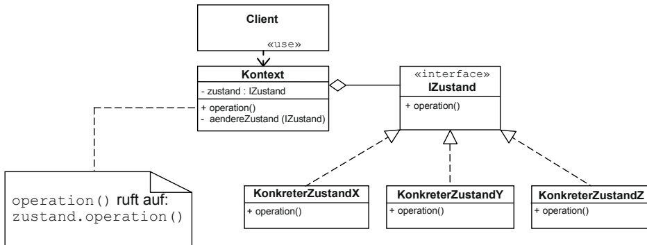
Bild 4-42 Klassendiagramm des Entwurfsmusters Zustand
