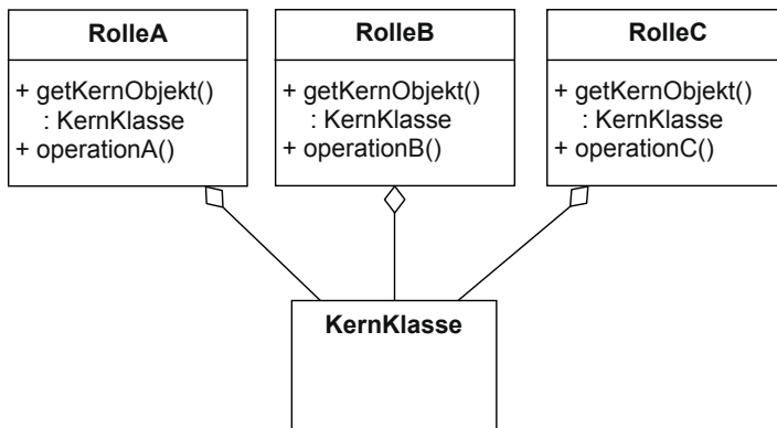
Bild 4-51 Klassendiagramm mit mehreren Rollen für eine Kernklasse
