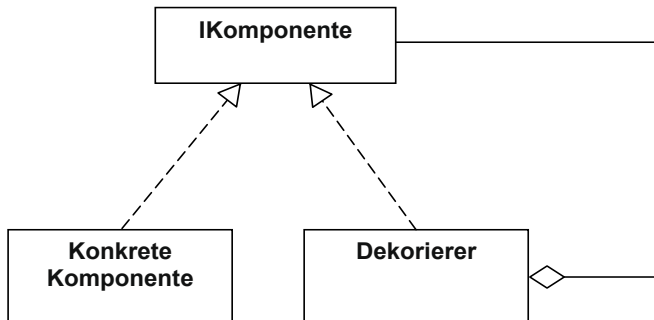
Bild 4-9 Dekorierer als Realisierung einer Schnittstelle
