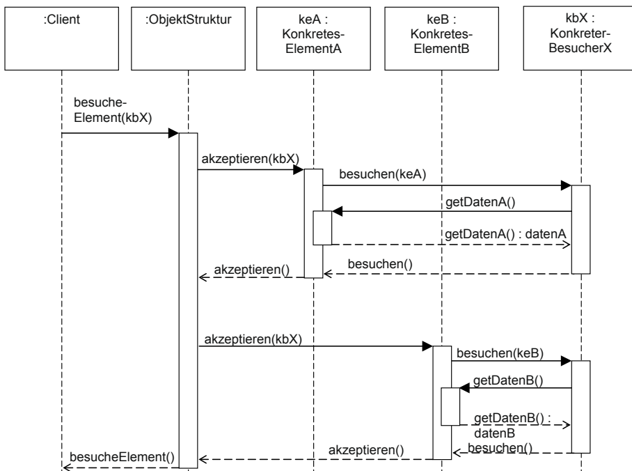
Bild 4-54 Sequenzdiagramm des Besucher-Musters
