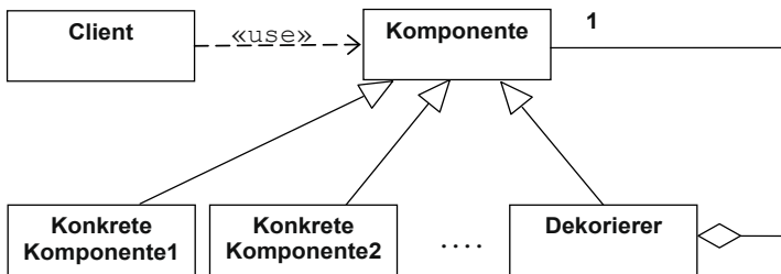
Bild 4-7 Klassendiagramm des Dekorierer-Musters
