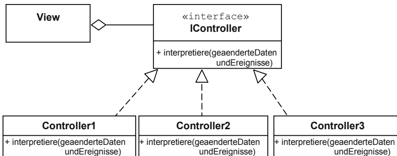
Bild 5-43 Klassendiagramm Strategie-Muster im MVC
