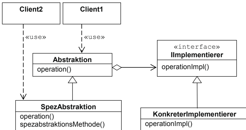
Bild 4-4 Klassendiagramm der Brücke mit dem Implementierer als Interface
