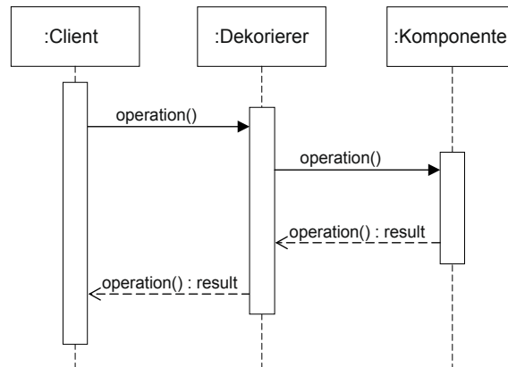
Bild 4-10 Sequenzdiagramm für die Dekoration einer Komponente
