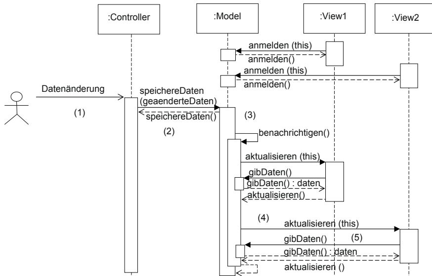
Bild 5-40 Sequenzdiagramm Aktualisierung des Model 113
