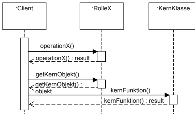
Bild 4-52 Sequenzdiagramm für eine Rollenoperation und eine Kernfunktion
