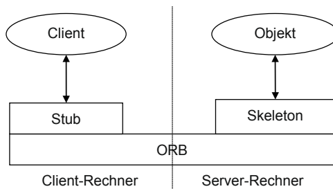
Bild 5-27 Struktur von CORBA
