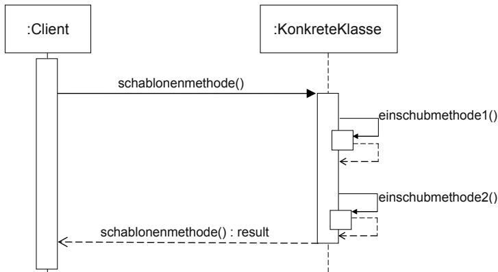
Bild 4-28 Sequenzdiagramm des Schablonenmethode-Musters
