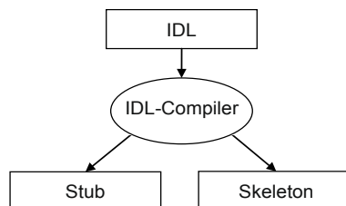
Bild 5-28 Erzeugung von Stub und Skeleton
