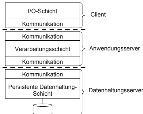
Bild 5-11 Modell der Drei-Schichten-Architektur mit Kommunikation
