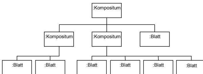
Bild 4-19 Struktur einer Teil-Ganzes-Hierarchie
