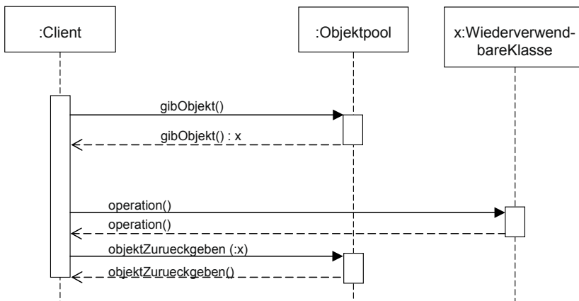
Bild 4-65 Abholen eines Objekts im Objektpool und Rückgabe
