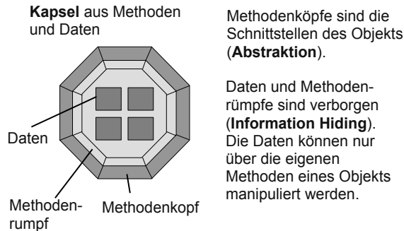
Bild 1-1 Daten und Methoden – die Bestandteile von Objekten
