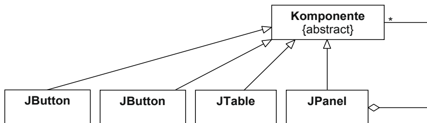
Bild 4-24 Klassendiagramm für eine Anwendung des Kompositum-Musters
