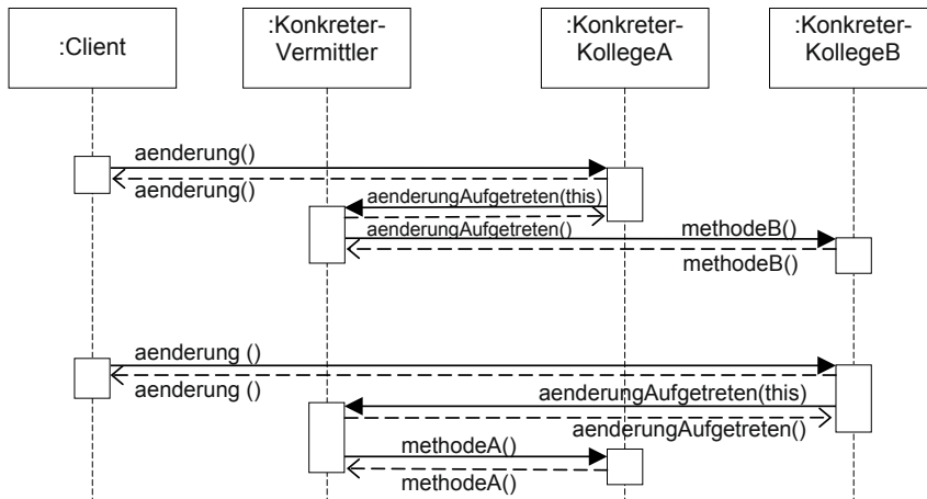
Bild 4-41 Sequenzdiagramm des Vermittler-Musters
