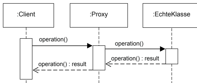
Bild 4-26 Sequenzdiagramm des Proxy-Musters
