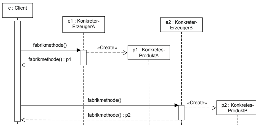
Bild 4-59 Sequenzdiagramm Fabrikmethode
