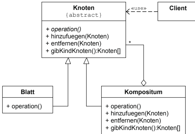
Bild 4-20 Klassendiagramm Kompositum
