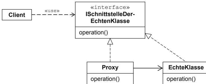
Bild 4-25 Klassendiagramm Proxy-Muster
