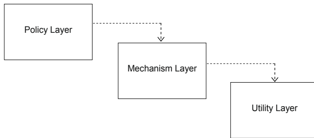
Bild 1-11 Einfache Ebenenstruktur
