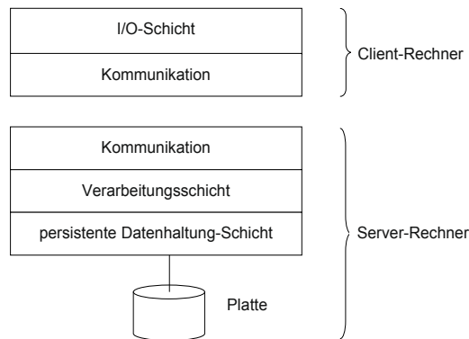
Bild 5-8 Beispiel für ein Schichtenmodell eines Client/Server-Rechners
