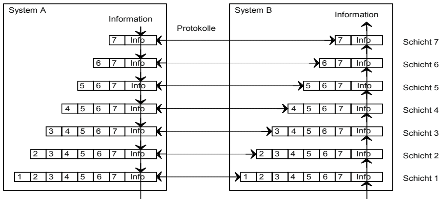
Bild 5-13 Protokollweg durch die OSI-Schichten
