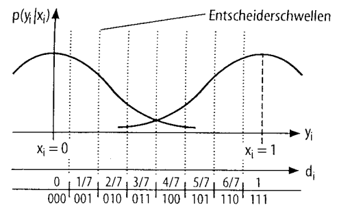
Abbildung 17a Softdecision
