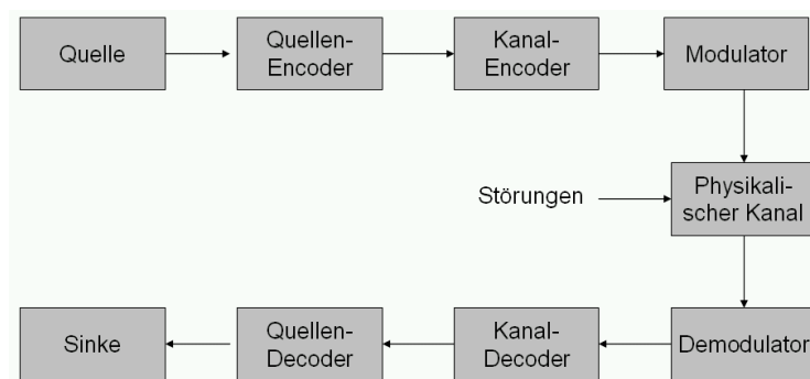
Abbildung 1 Übertragungsstrecke
