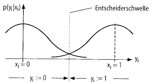
Abbildung 16a Harddecision
