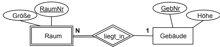
Abb. 2-26: Existenzabhängige Entitätstypen
