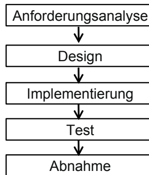
Abb. 2-1: Einfacher Software-Entwicklungsprozess
