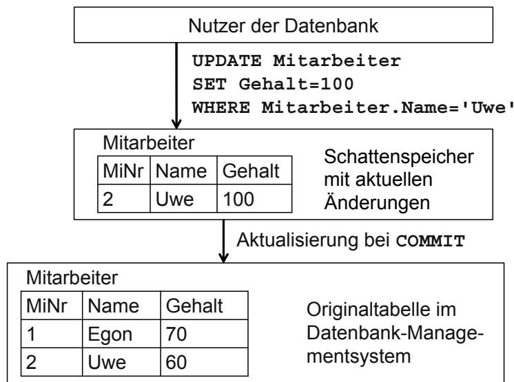
Abb. 10-1: Schattenspeicher-Verfahren
