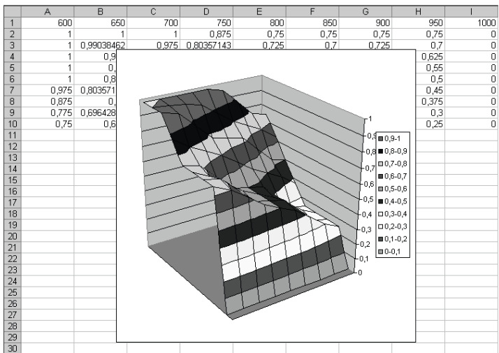
Abbildung 11-14: Berechnetes Kennfeld
