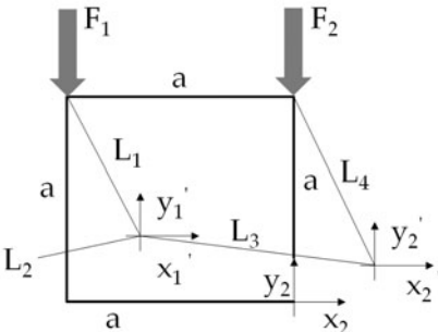
Abbildung 10-7: Verschiebung des 2. Knotens
