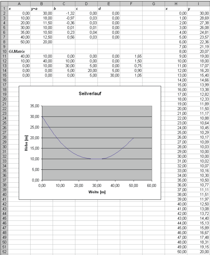
Abbildung 4-7: Durch kubische Splines ermittelter Seilverlauf
