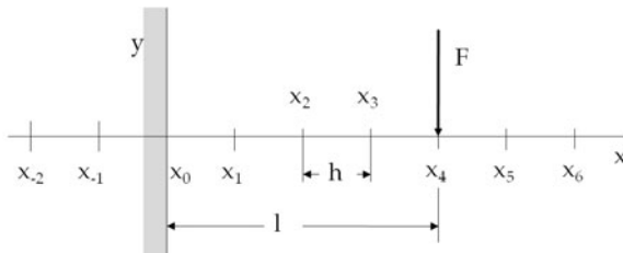
Abbildung 6-7: Einseitig eingespannter Biegeträger
