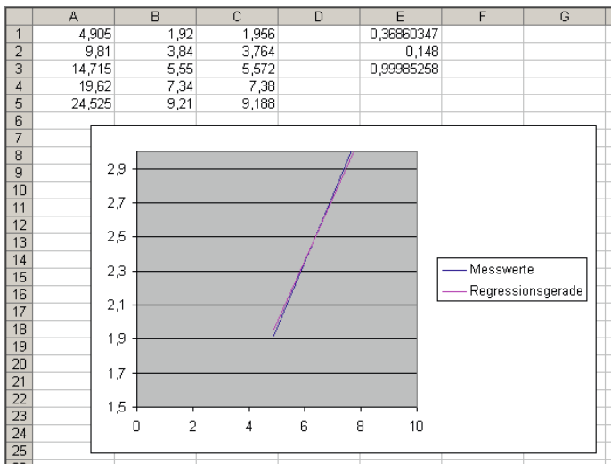
Abbildung 8-10: Bestimmung der Federkonstanten aus den Beispieldaten
