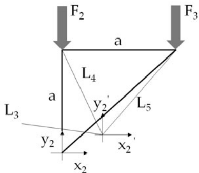
Abbildung 10-8: Der Endstab
